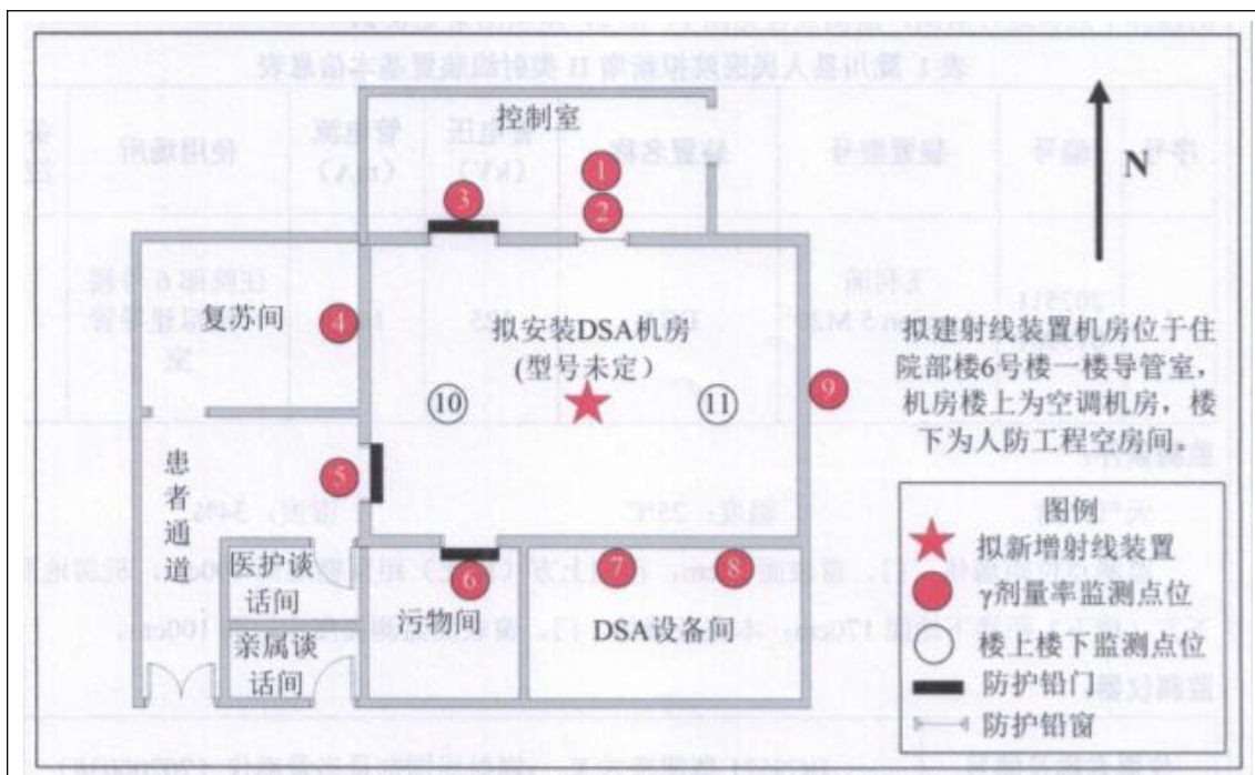
图 8-1 拟新增II类射线装置机房区域周围 X-γ辐射剂量率监测点示意图
