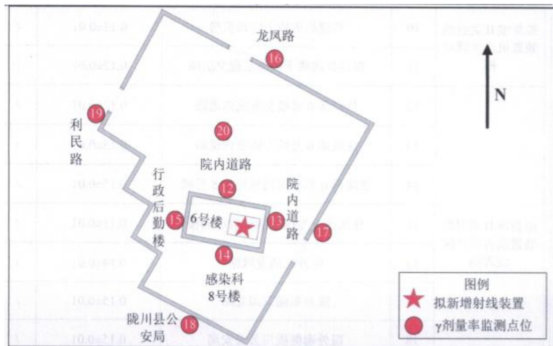
图 8-2 拟新增II类射线装置院内区域周围 X-γ辐射剂量率监测点示意图
