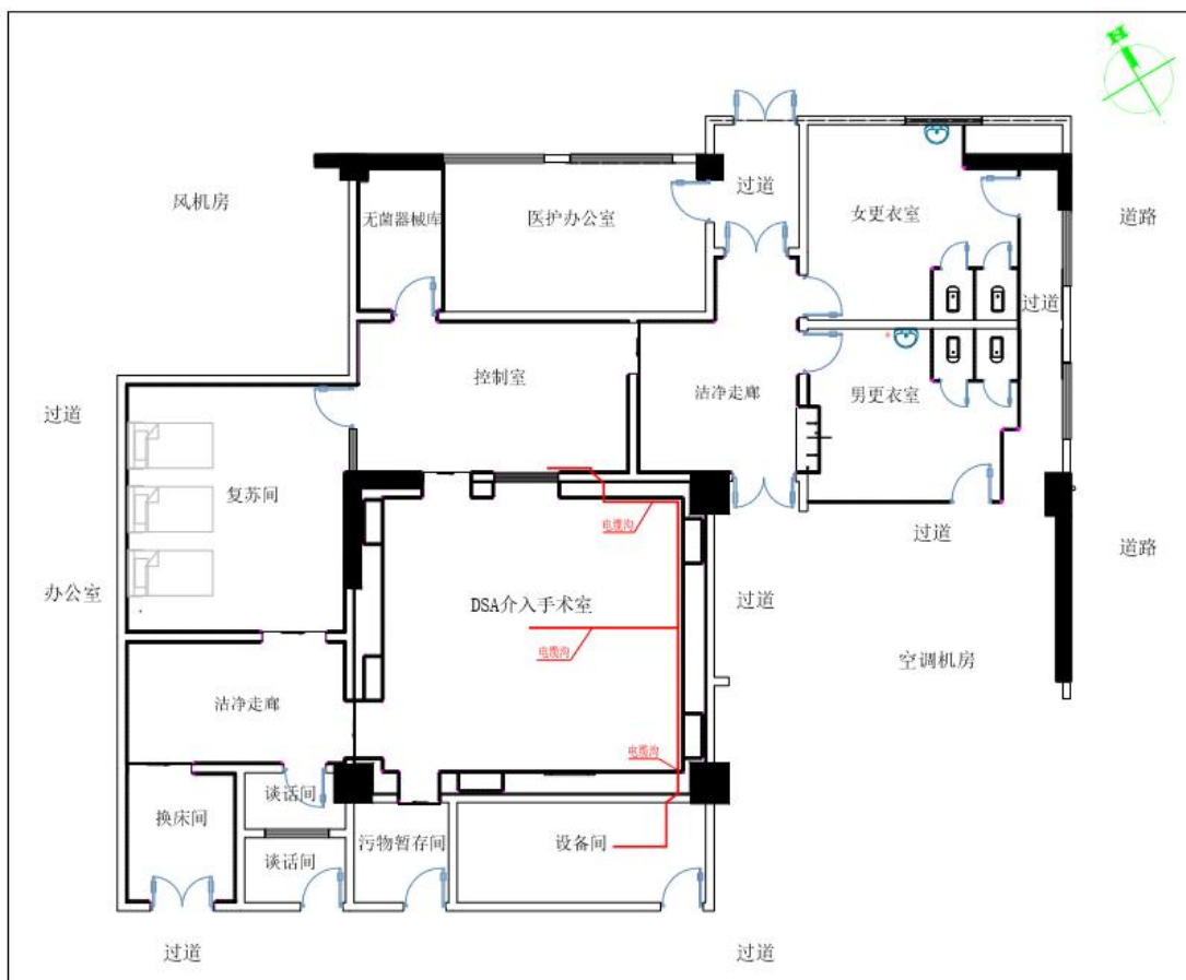
图 10-4 电缆沟平面布置图
