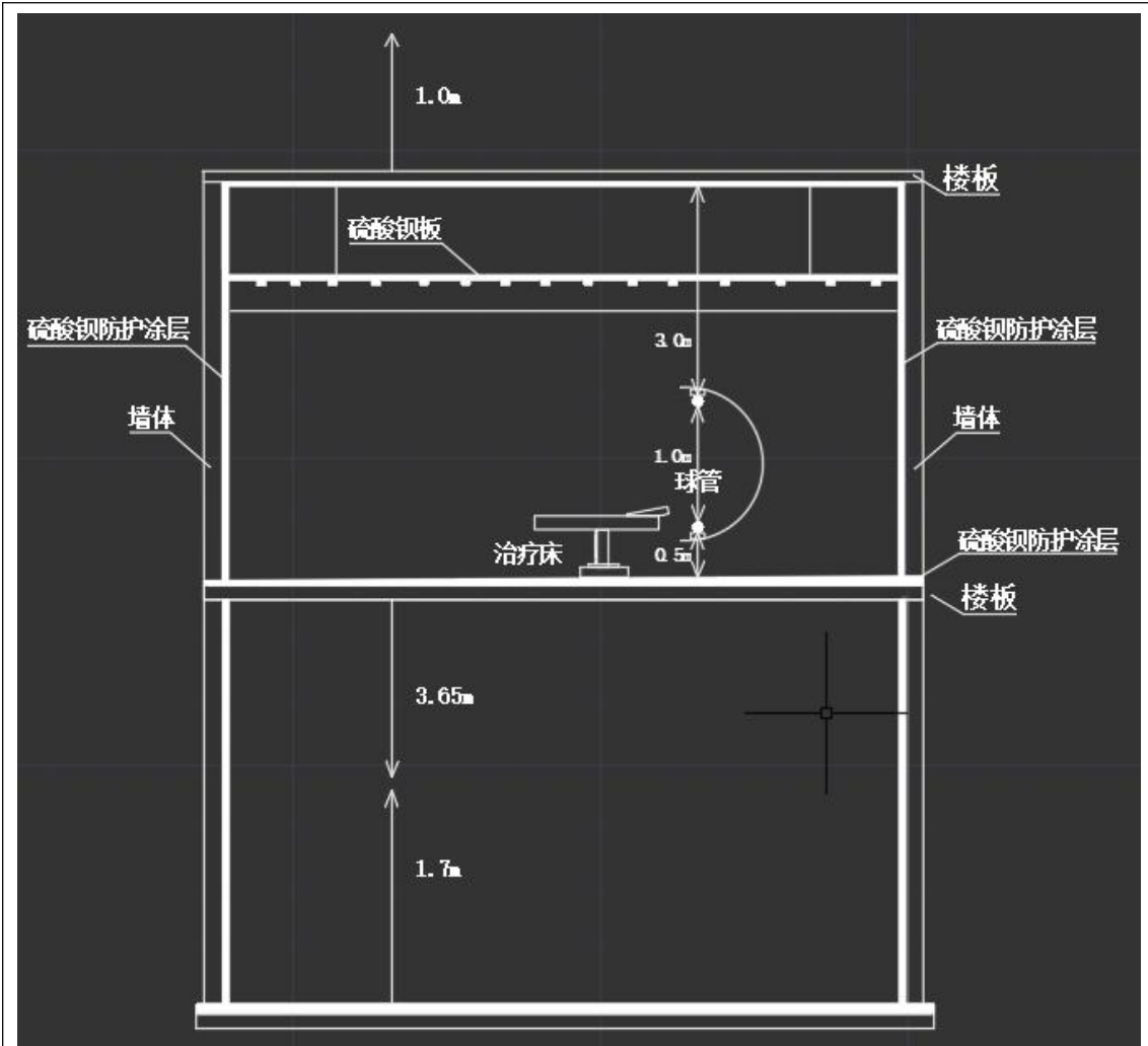
图 11-3 DSA 手术室楼上、楼下注点位置
