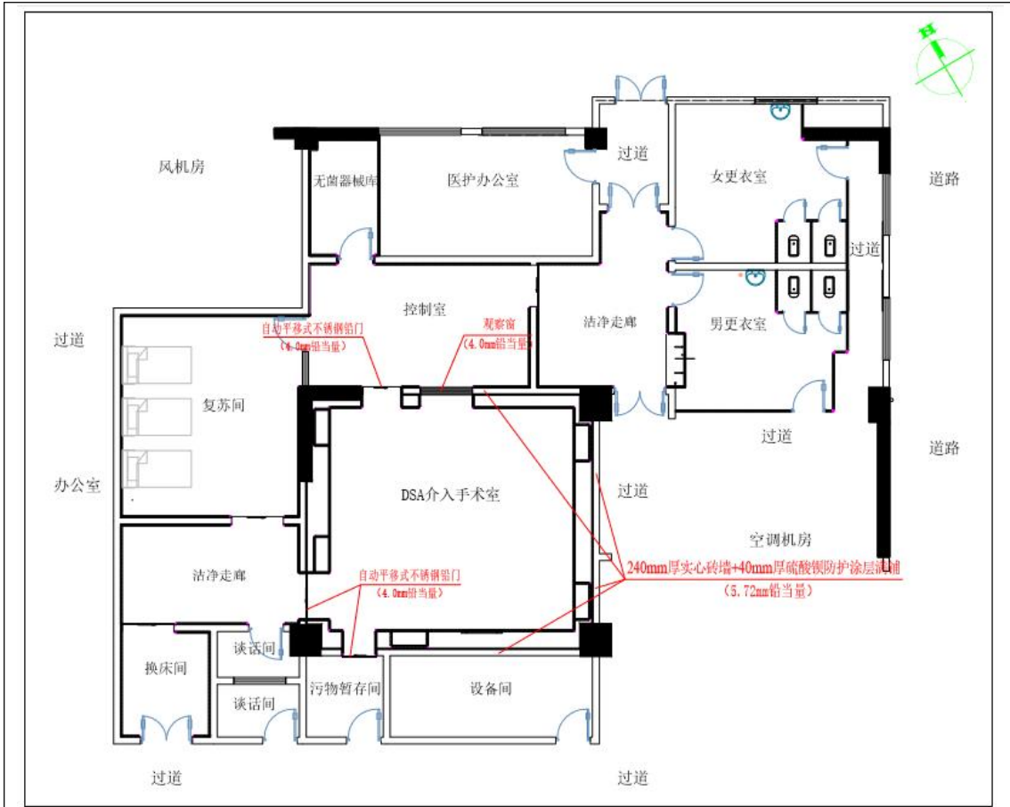
图 10-1 机房屏蔽防护平面图
