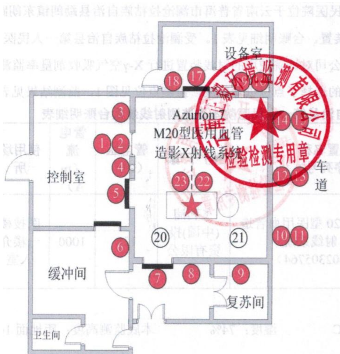
图 11-1 类比项目介入室周围监测布点示意图
