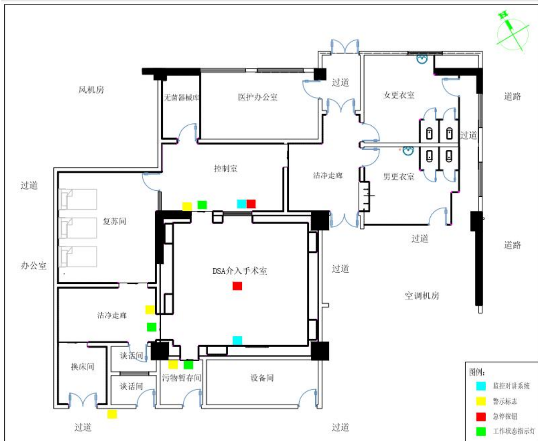
图 10-3 辐射安全措施平面布置图
