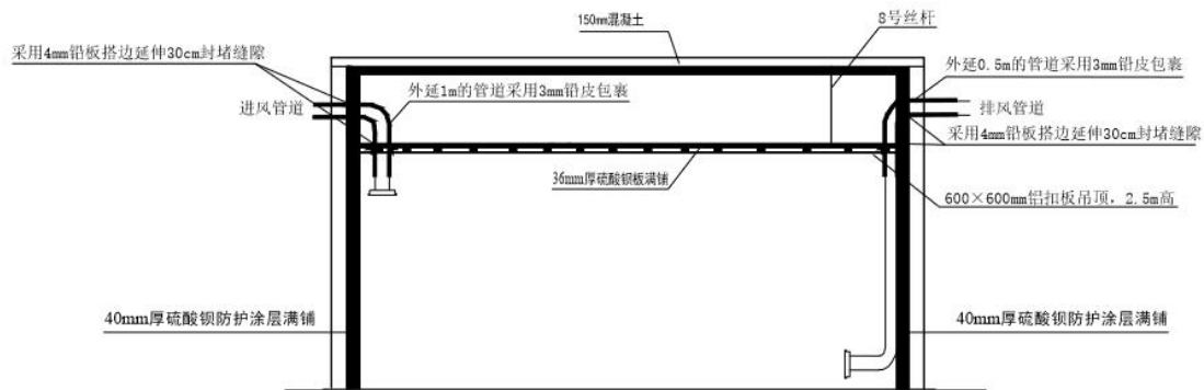
图 10-6 通风管道剖面图
