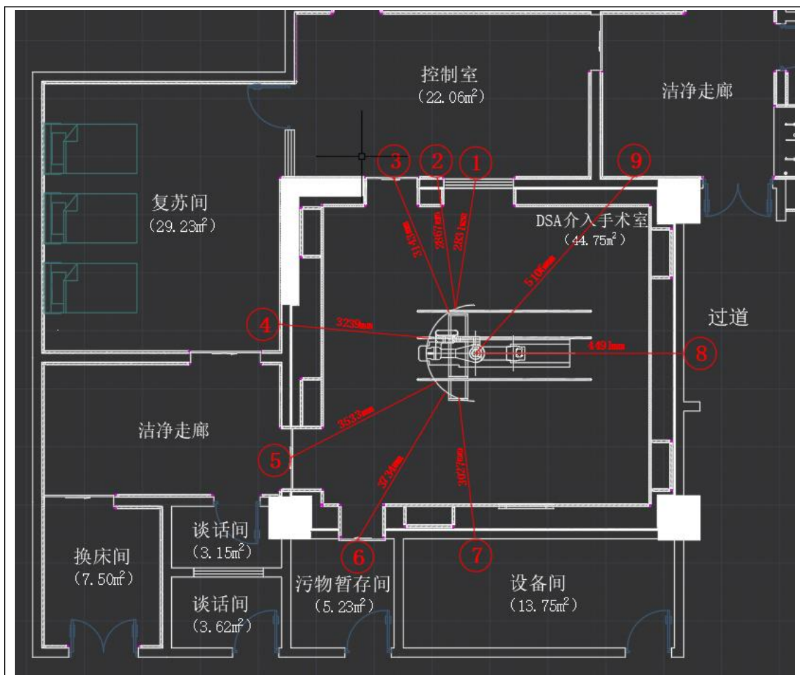
图 11-2 DSA 手术室外四周各关注点位置
