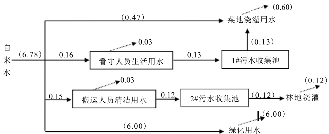
图 4-3 水平衡图 (m 3 /d)
